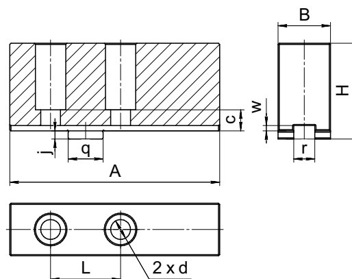
Кулачок реверсивный
