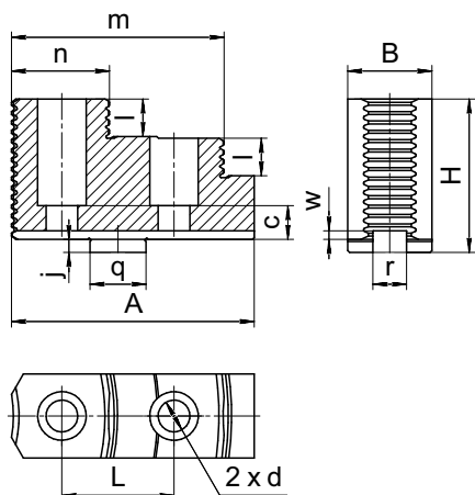
Кулачок накладной мягкий
