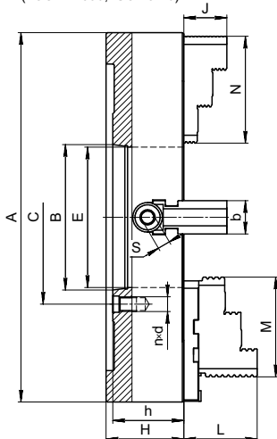
Тип крепления 2 «J» (ГОСТ 12593; ISO 702-3)
